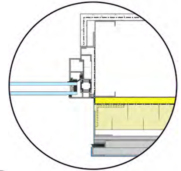
Jamb Detail
